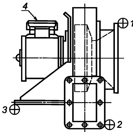
Рисунок 7 — Рекомендуемые точки измерений для осевого вентилятора
