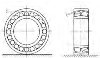
Рис. 1. Проверка зазора подшипника на верстаке.
